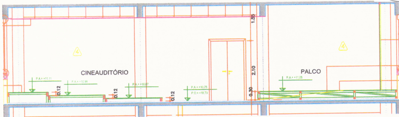
1 CORTE B B' ESCALA 1/75
